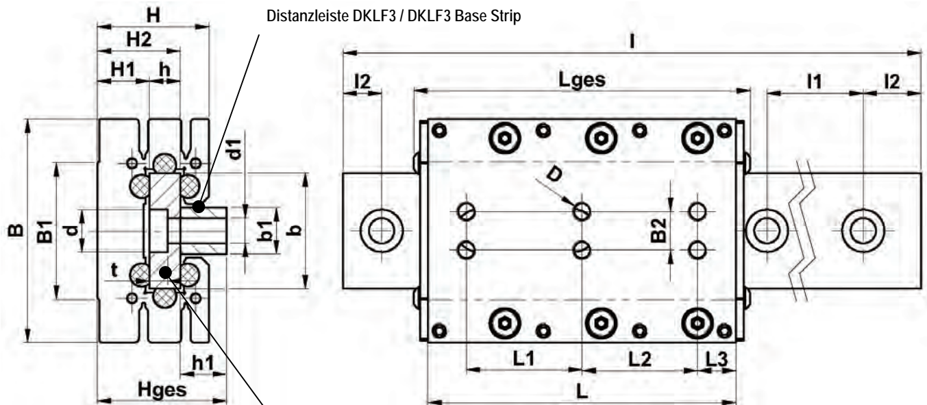
Führungsschiene DKLF3/80-20 DKLF3/80-20 Guide rail
