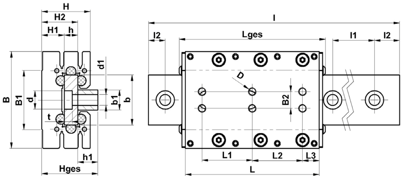
Abmessung Führungsschlitten DKLF3 Dimensions of DKLF3 Carriages
